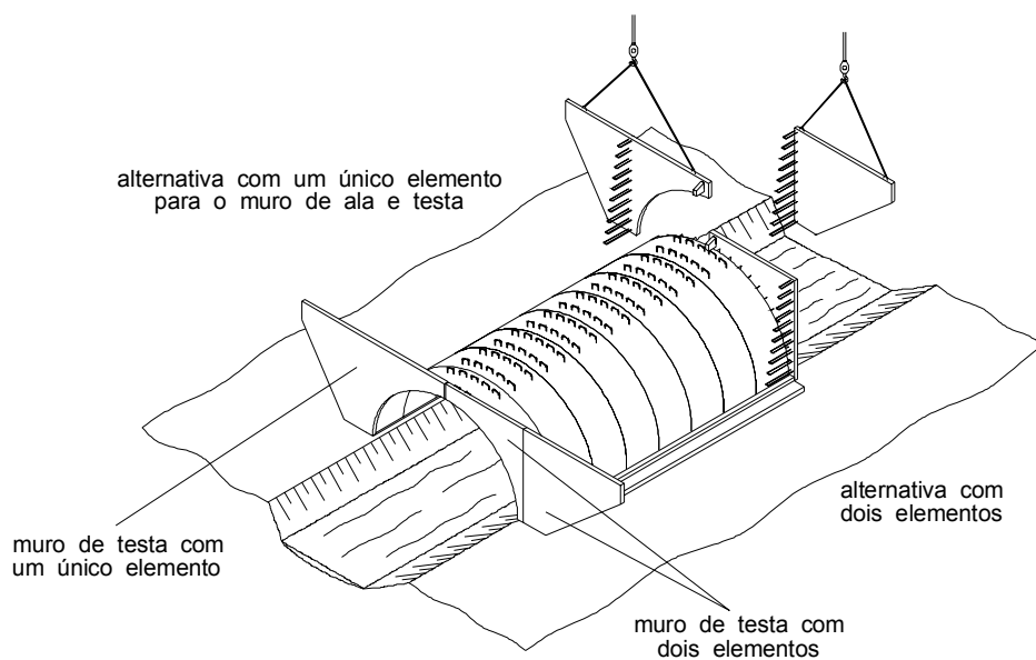
a) colocação dos elementos correspondentes aos muros (esquerda com um único elemento e a direita com dois elementos)
