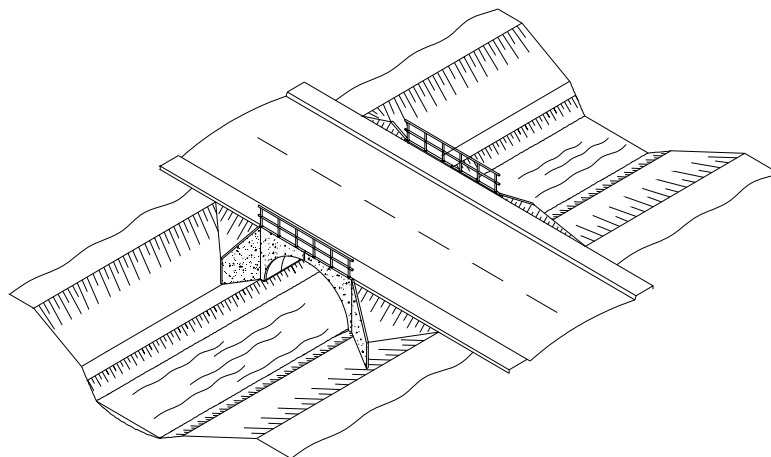
e) execução do guarda-corpo, aterro, passeio e pavimentação (término da construção)
