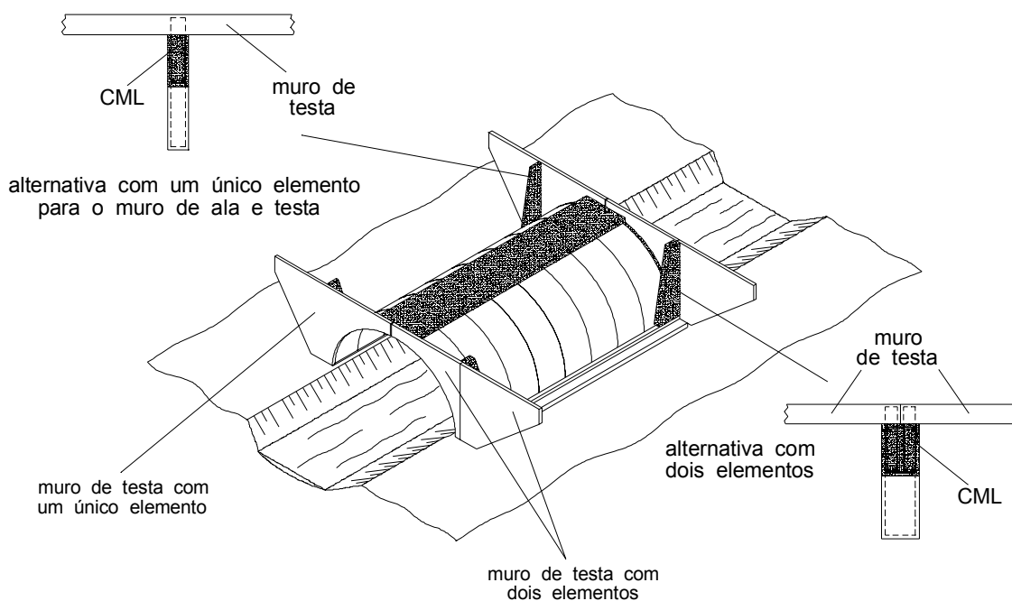
b) colocação da armadura complementar e das fôrmas; execução da concretagem das partes de concreto moldado no local (término da estrutura)
