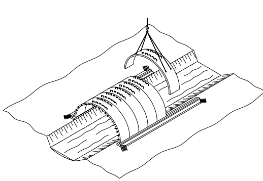
a) colocação das abóbodas pré-moldadas sobre fundação de concreto moldado no local
