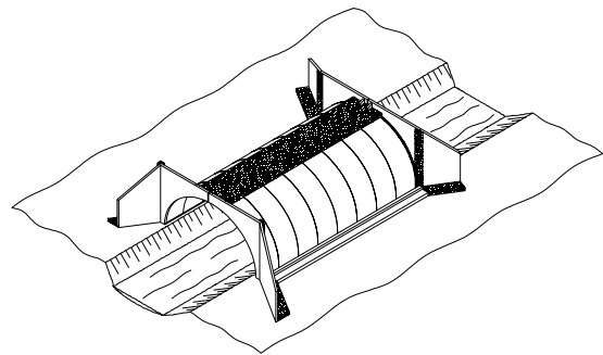
d) colocação da armadura complementar e das fôrmas; moldagem das partes de concreto moldado no local (término da estrutura)
