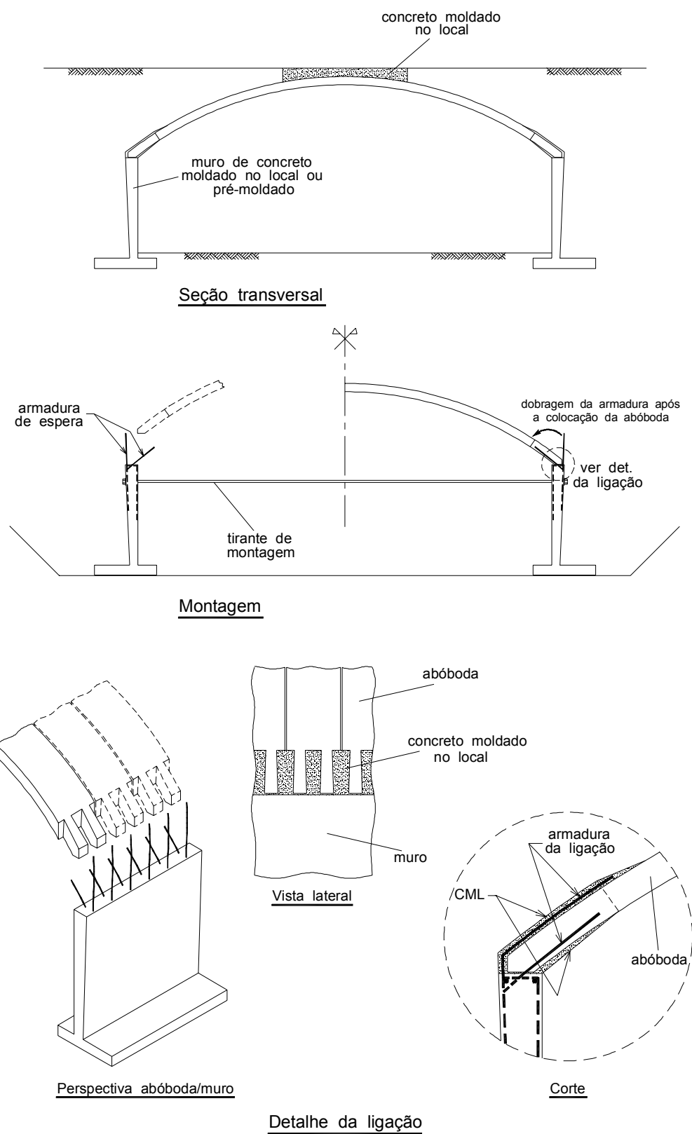
Figura 13 - Pontilhão em "pseudo" pórtico
