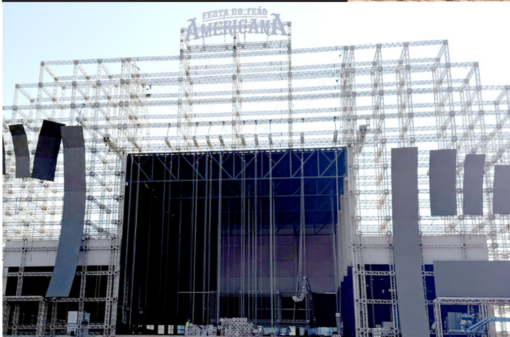
Palco da Festa do Peão, em Americana, em fase de execução
